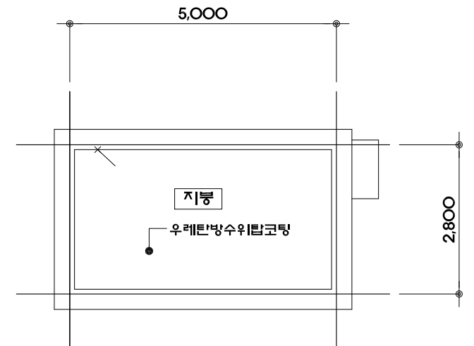
옥탑지붕 평면도 scale:1/100
